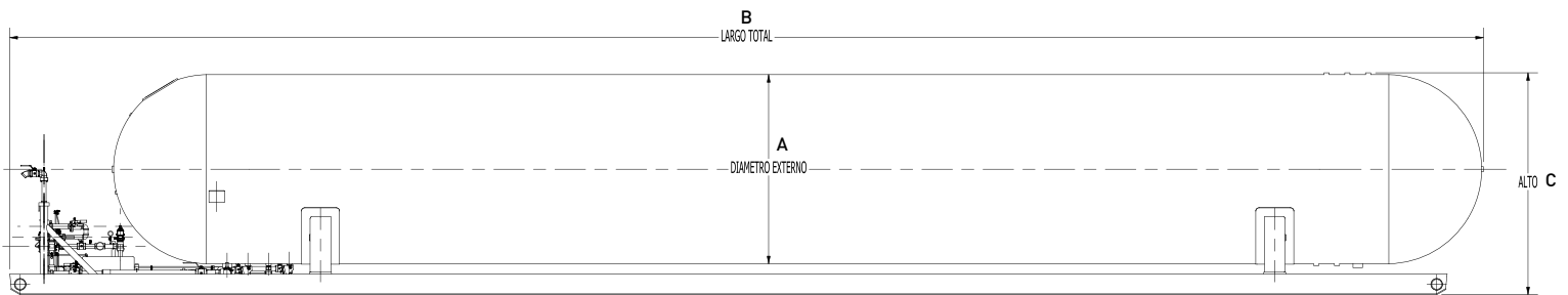
VISTA LATERAL
